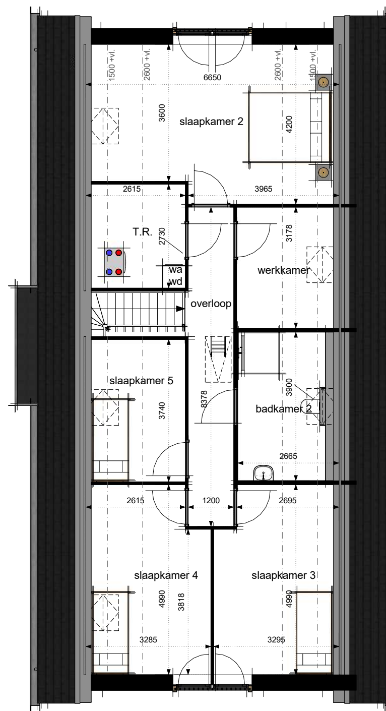
verdieping
